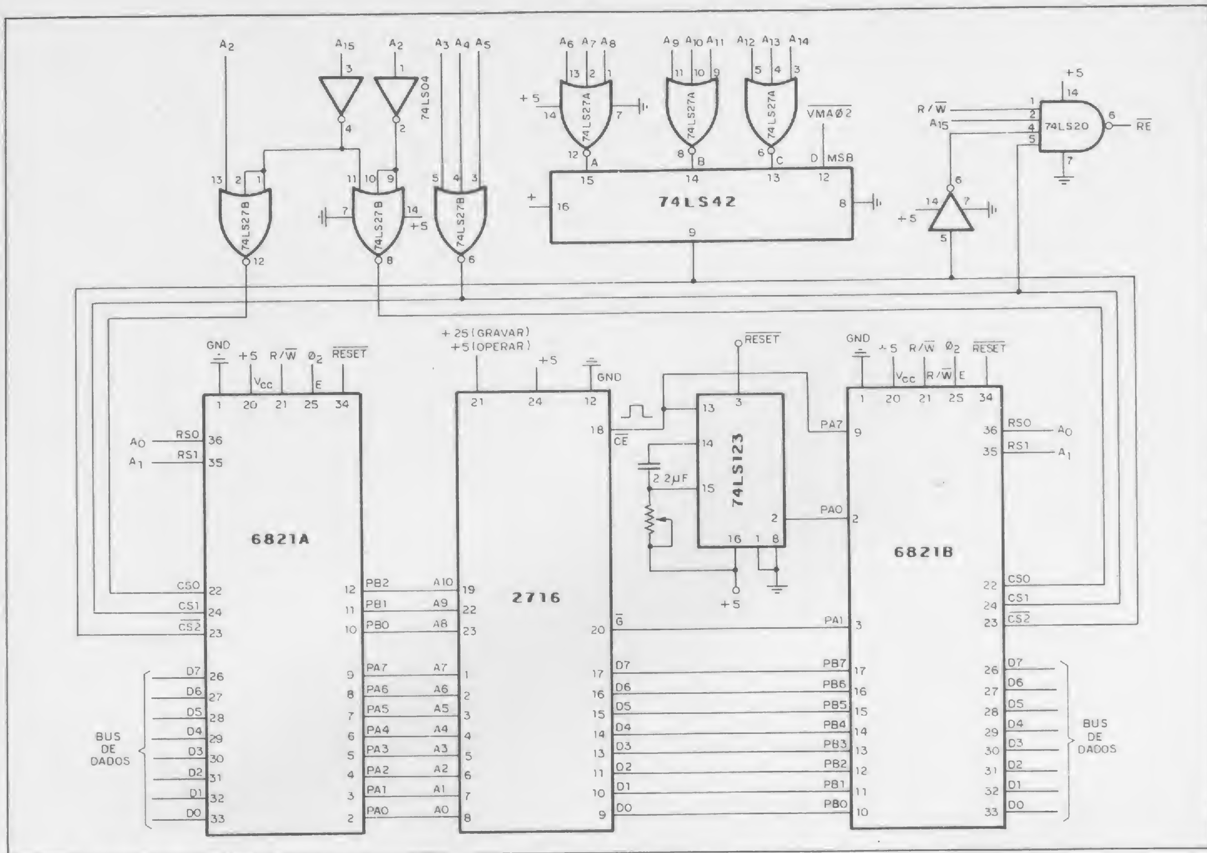
Figura 1 - O circuito de gravação/verificação.
